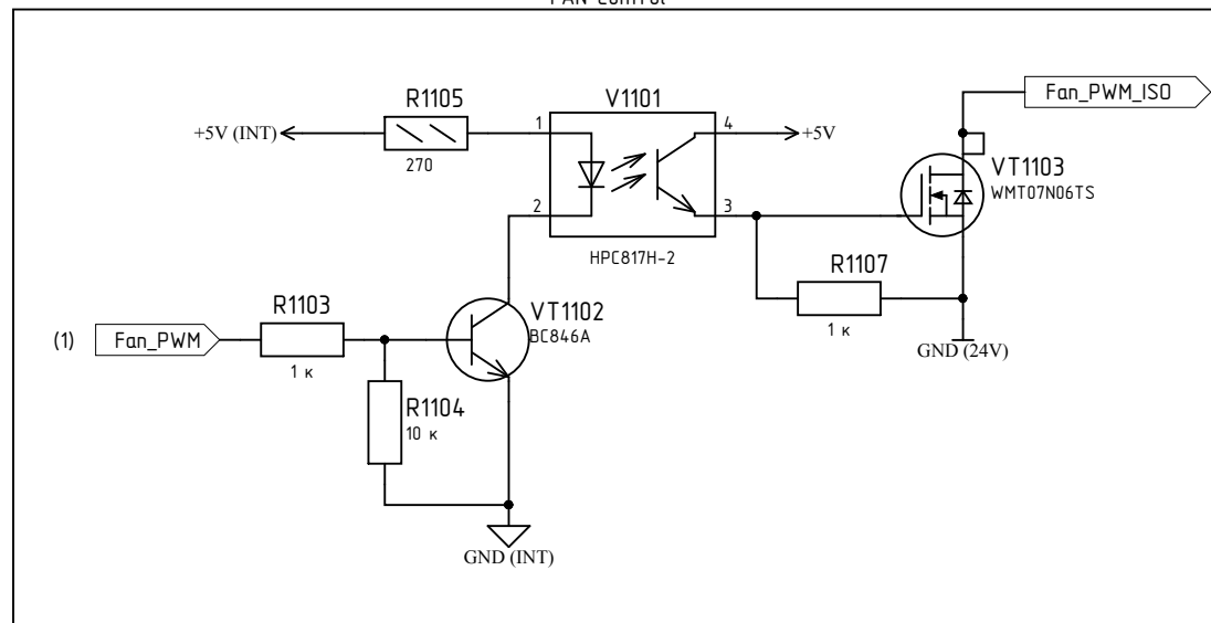
FAN Control
