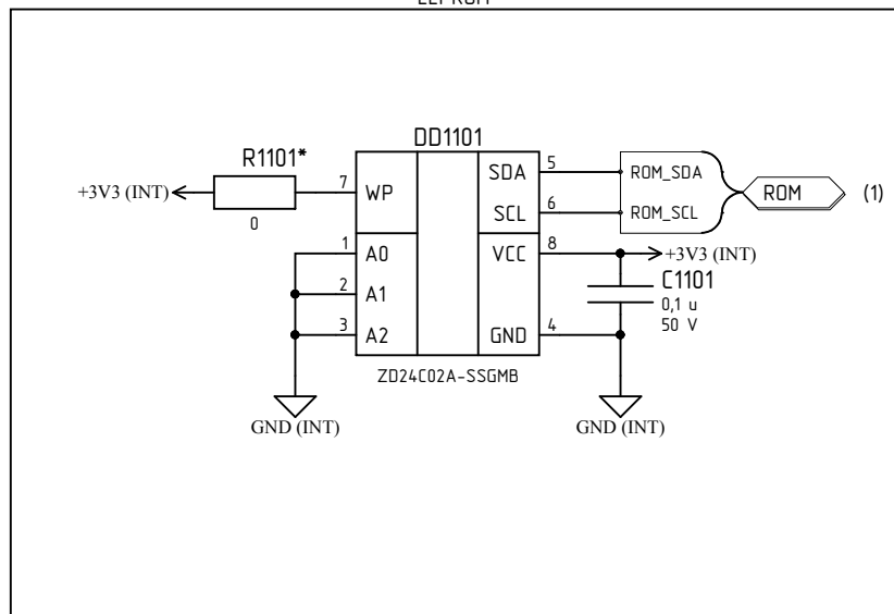
EEPROM
